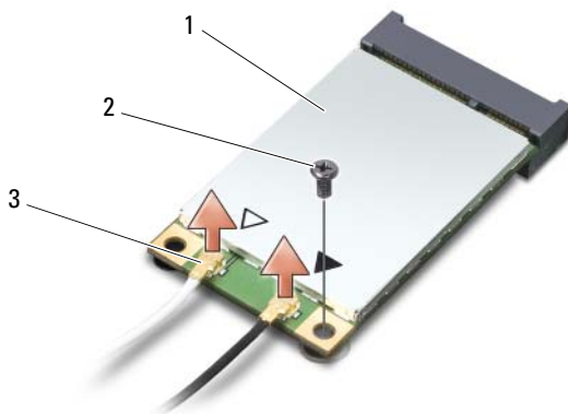
1 scheda WWAN 2 vite M2 x 3 mm 3 connettori dei cavi dell'antenna (2)
