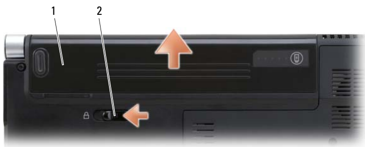
1 batteria 2 chiusura a scatto della batteria
